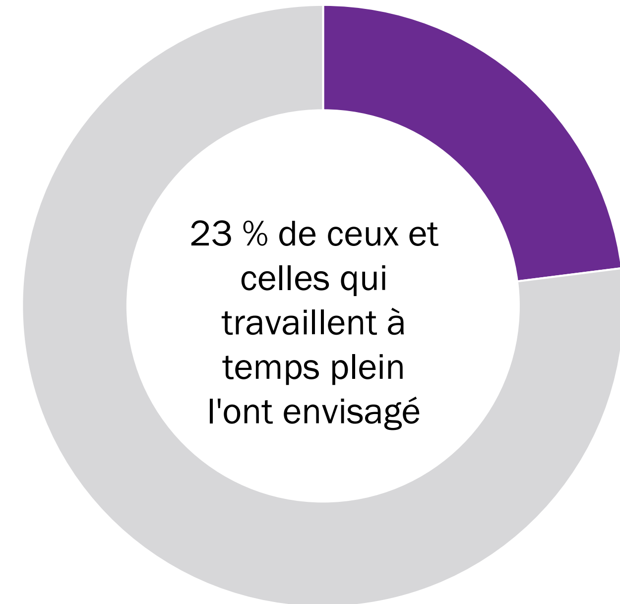
Base : 1 010
