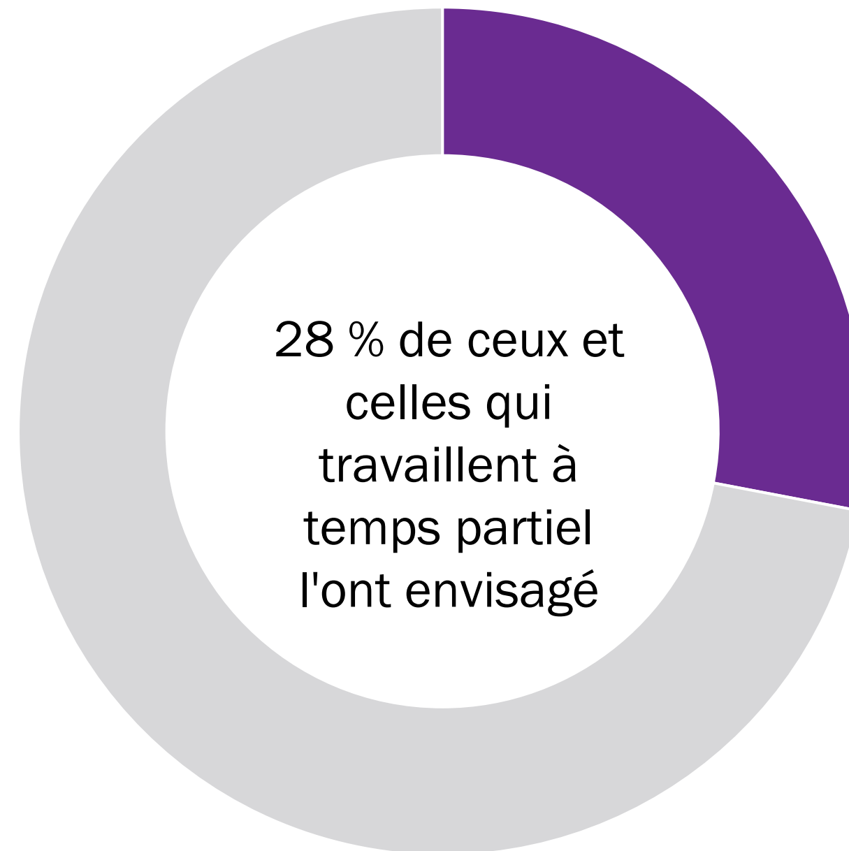
Base : 2 019
