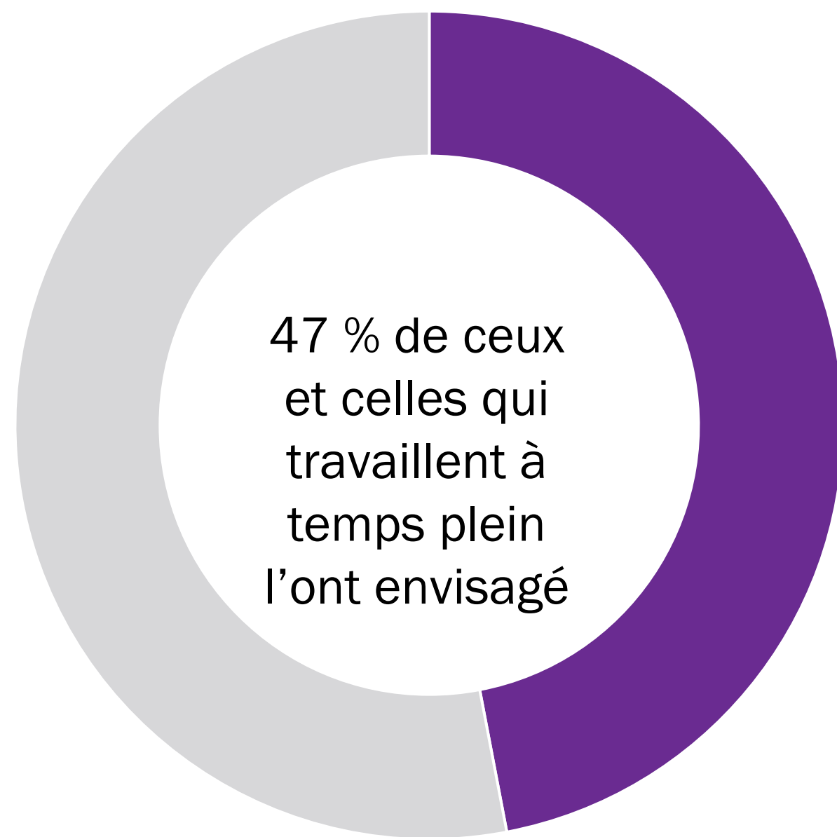
Base : 322
